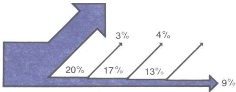
Рис. 2. Распределение энергии топлива при движении автомобиля.
