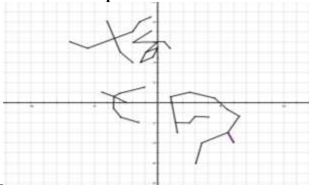
карта осеннего неба
